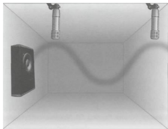
Рис. 84. два микрофона, снимающие звук в фазе.
